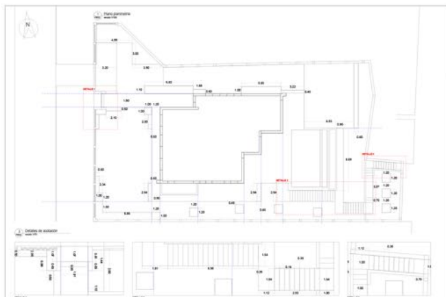
02. PLANO PLANIMÉTRICO
