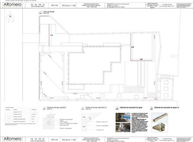
07. PLANO DRENAJE
